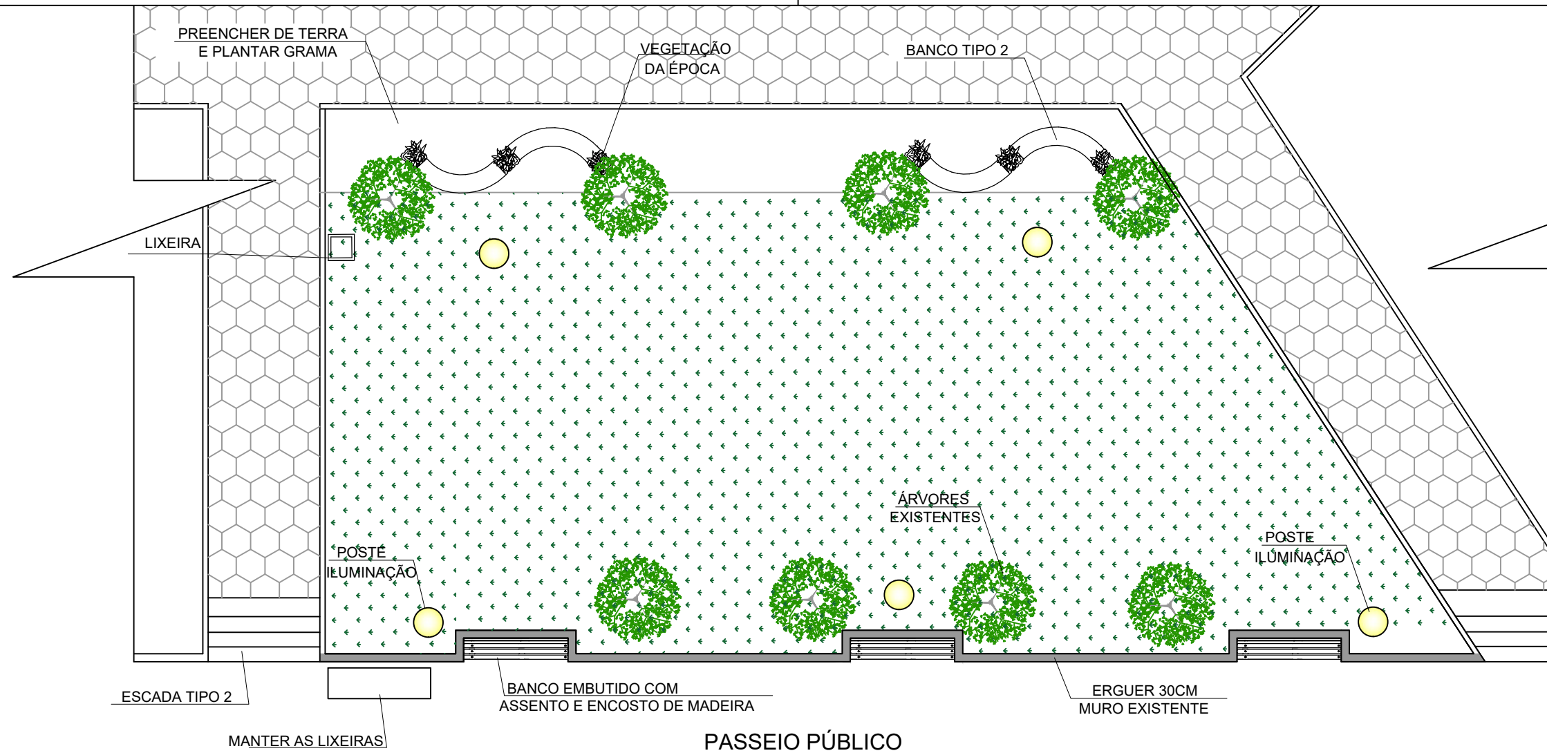
1 CANTEIRO 2 - PLANTA BAIXA
